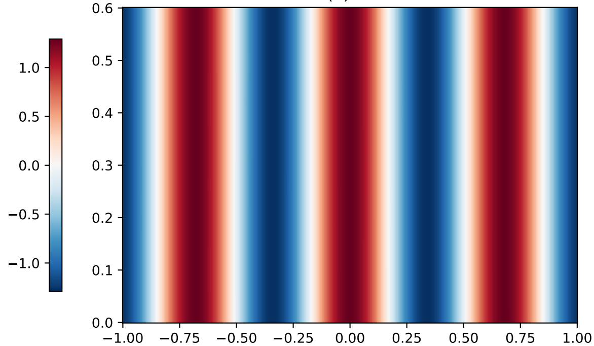
Re(u) PINN
